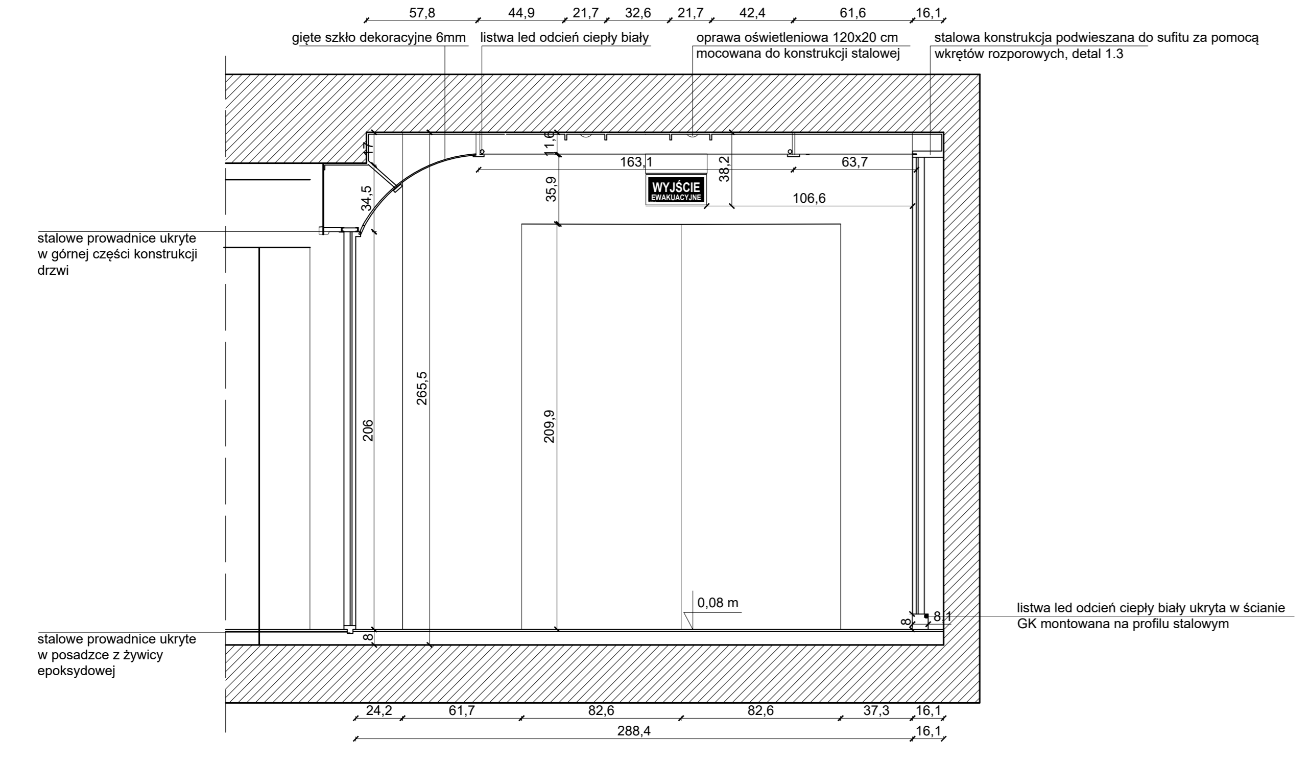
PRZEKRÓJ B-B
